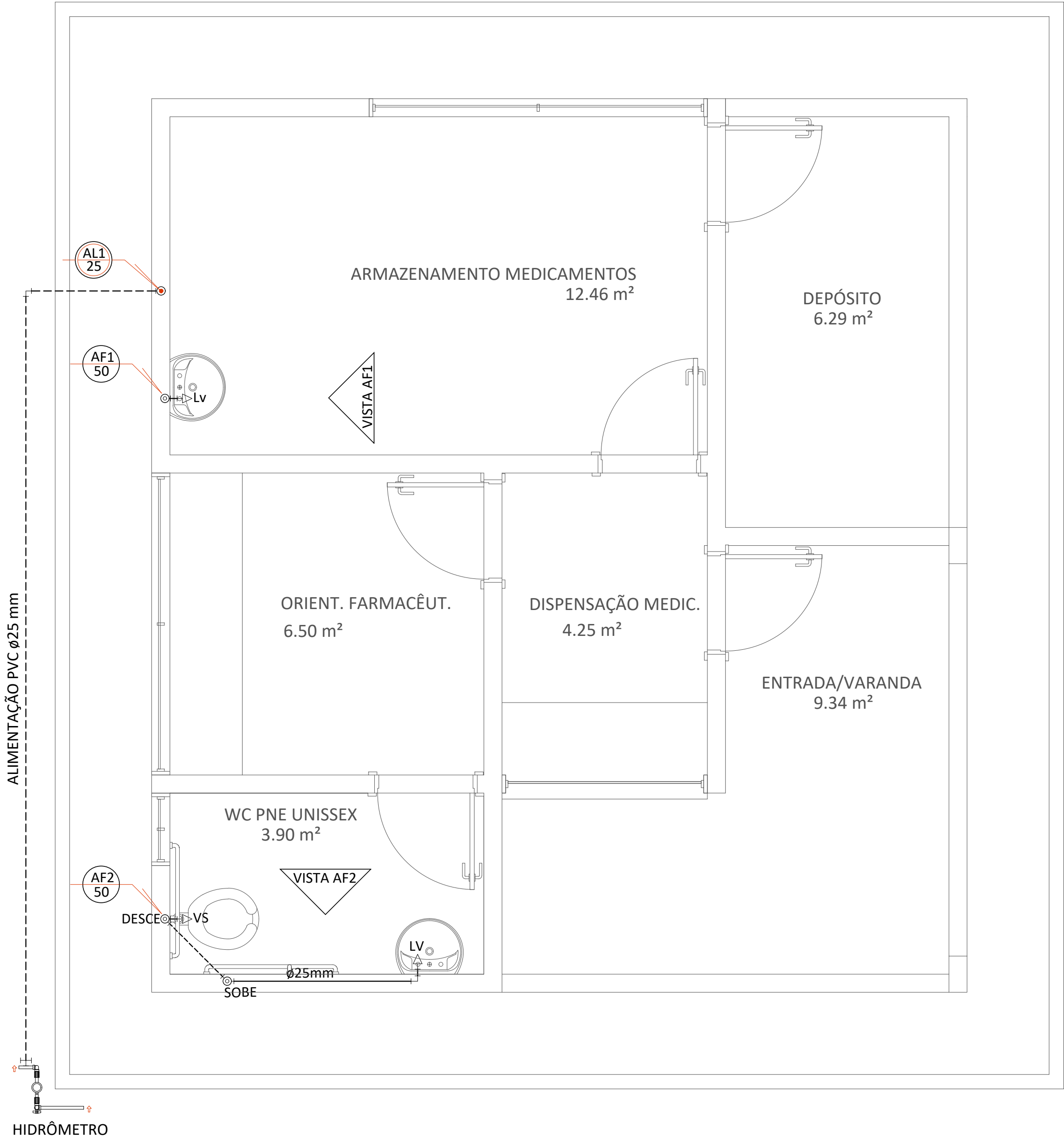
PLANTA BAIXA - INSTALAÇÃO HIDRÁULICA
