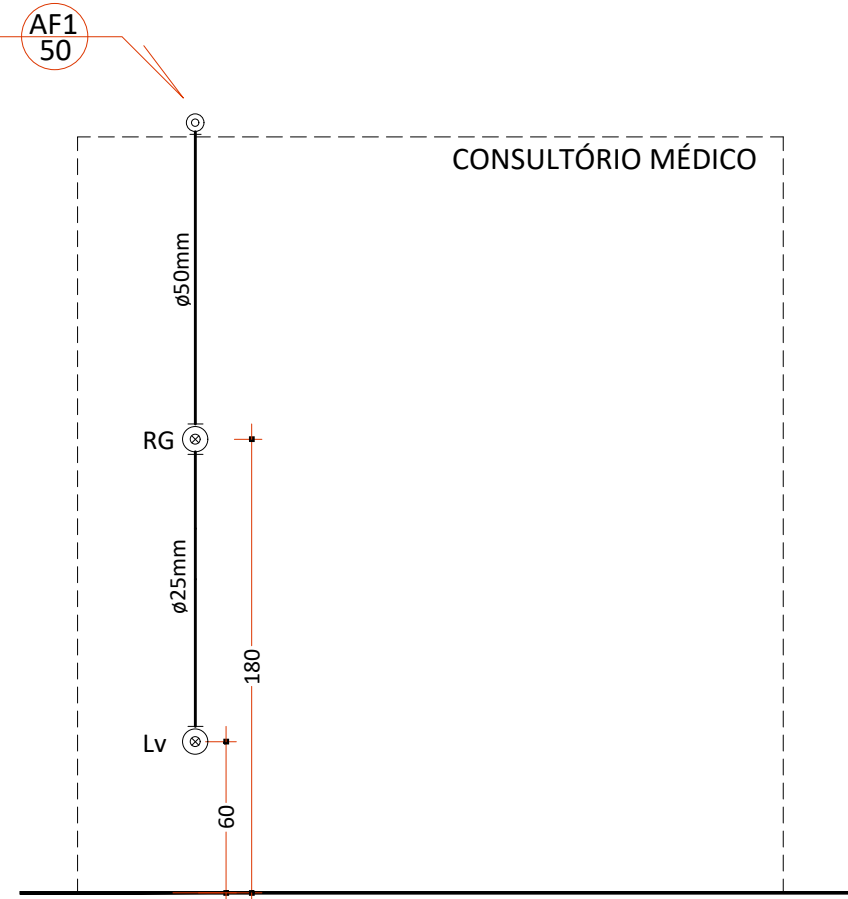
VISTA 1 Escala 1:30
