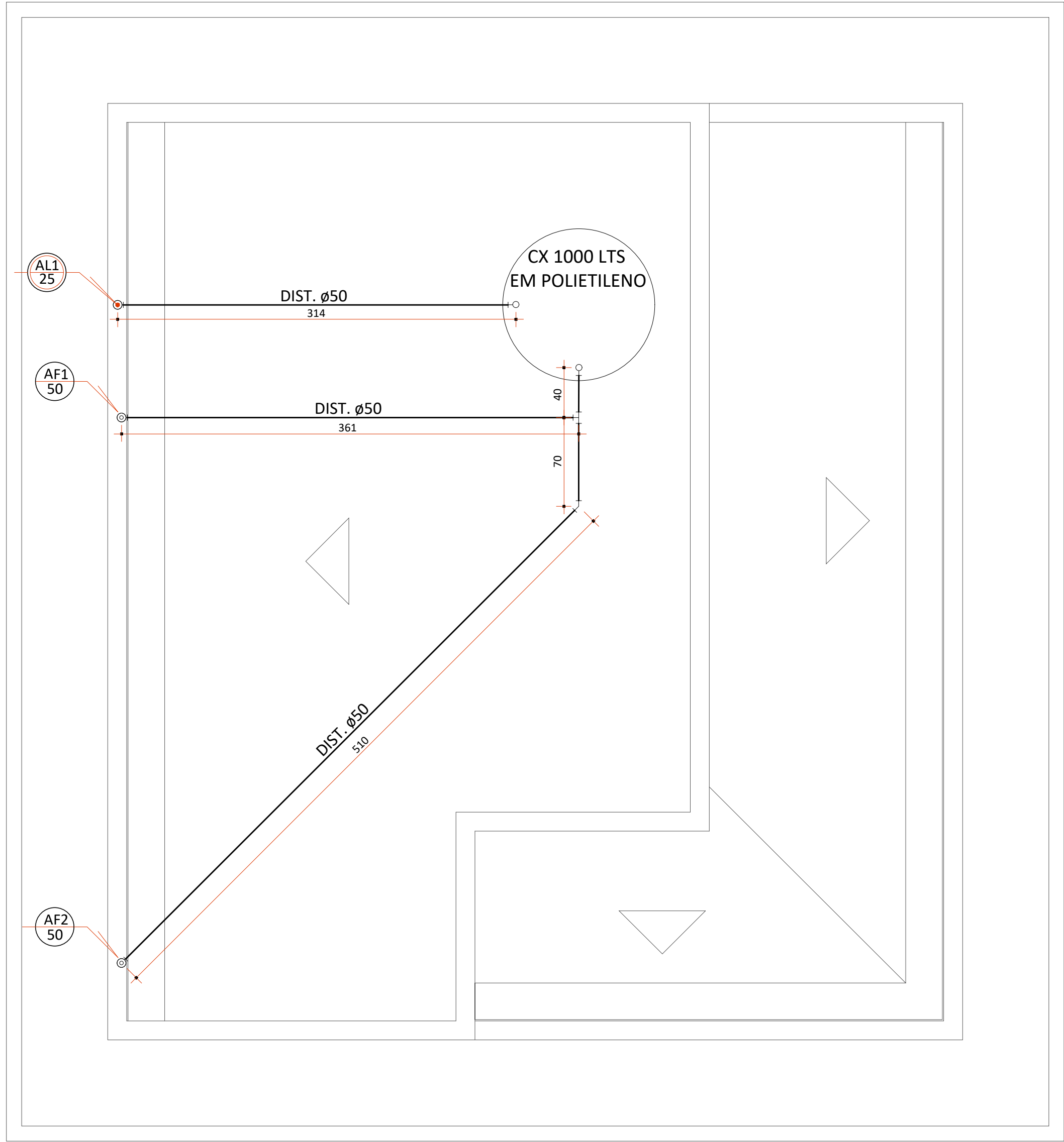
PLANTA COBERTURA - INSTALAÇÃO HIDRÁULICA
