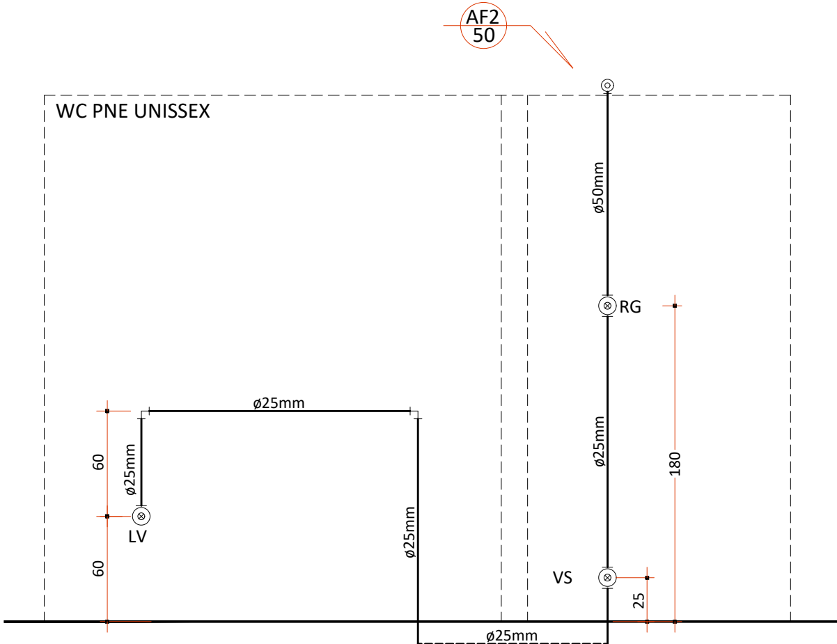
VISTA 2 Escala 1:30
