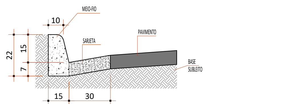
DETALHE - MEIO-FIO E SARIETA
