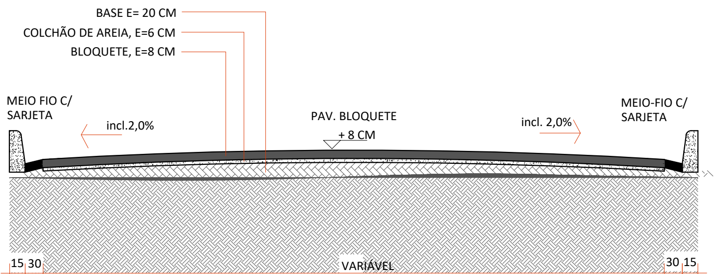
DETALHE - PERFIL DO PAVIMENTO
