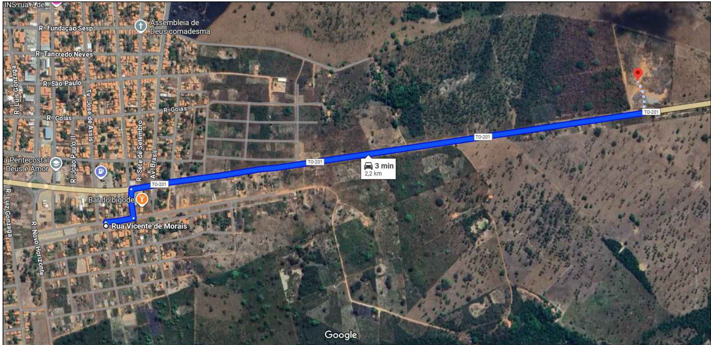
MAPA DE PERCURSO DA JAZIDA/BOTA-FORA AO CENTRO DE MASSA DA PAVIMENTAÇÃO - (DMT = 2,2 KM)
