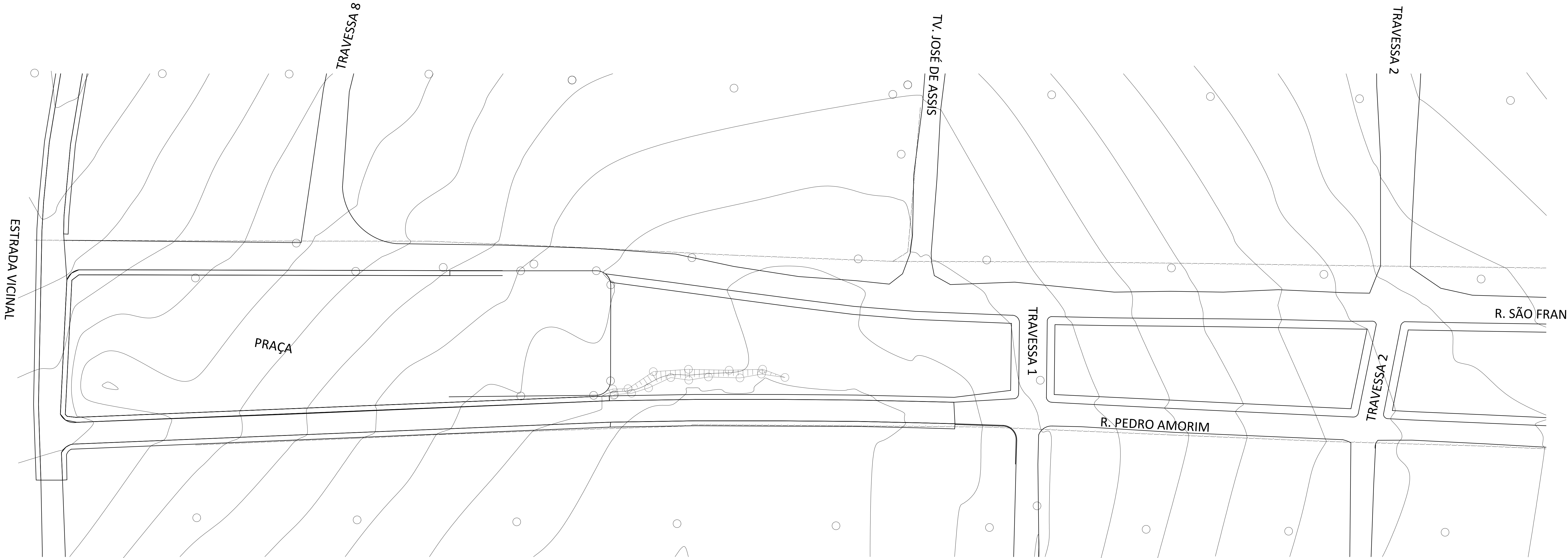
LEVANTAMENTO TOPOGRÁFICO - RUAS SÃO FRANCISCO, PEDRO AMORIM, TRAVESSA 1 E TRAVESSA 2
