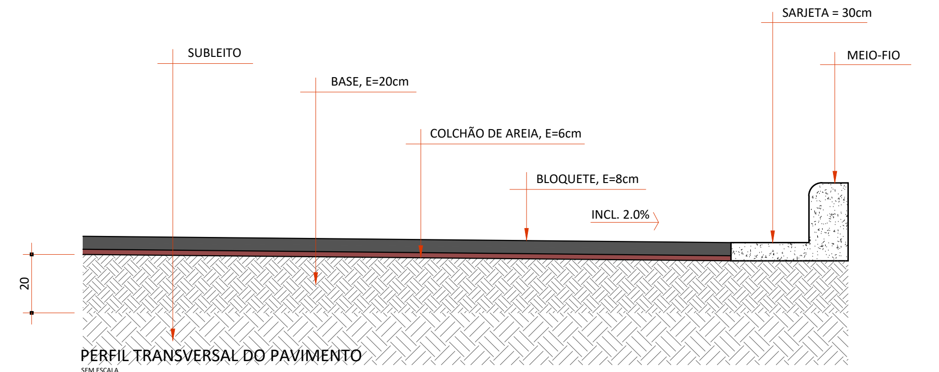
PERFIL TRANSVERSAL DO PAVIMENTO
